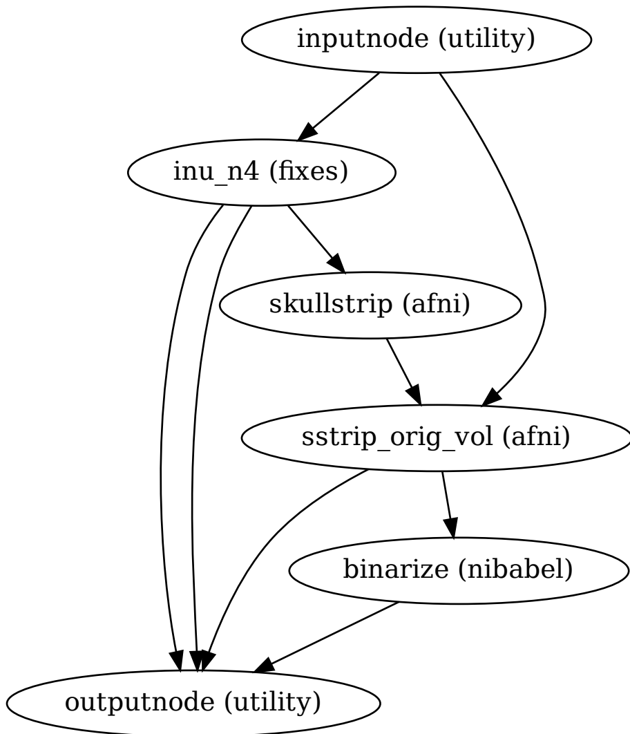
AFNISKullStripWorkflow
