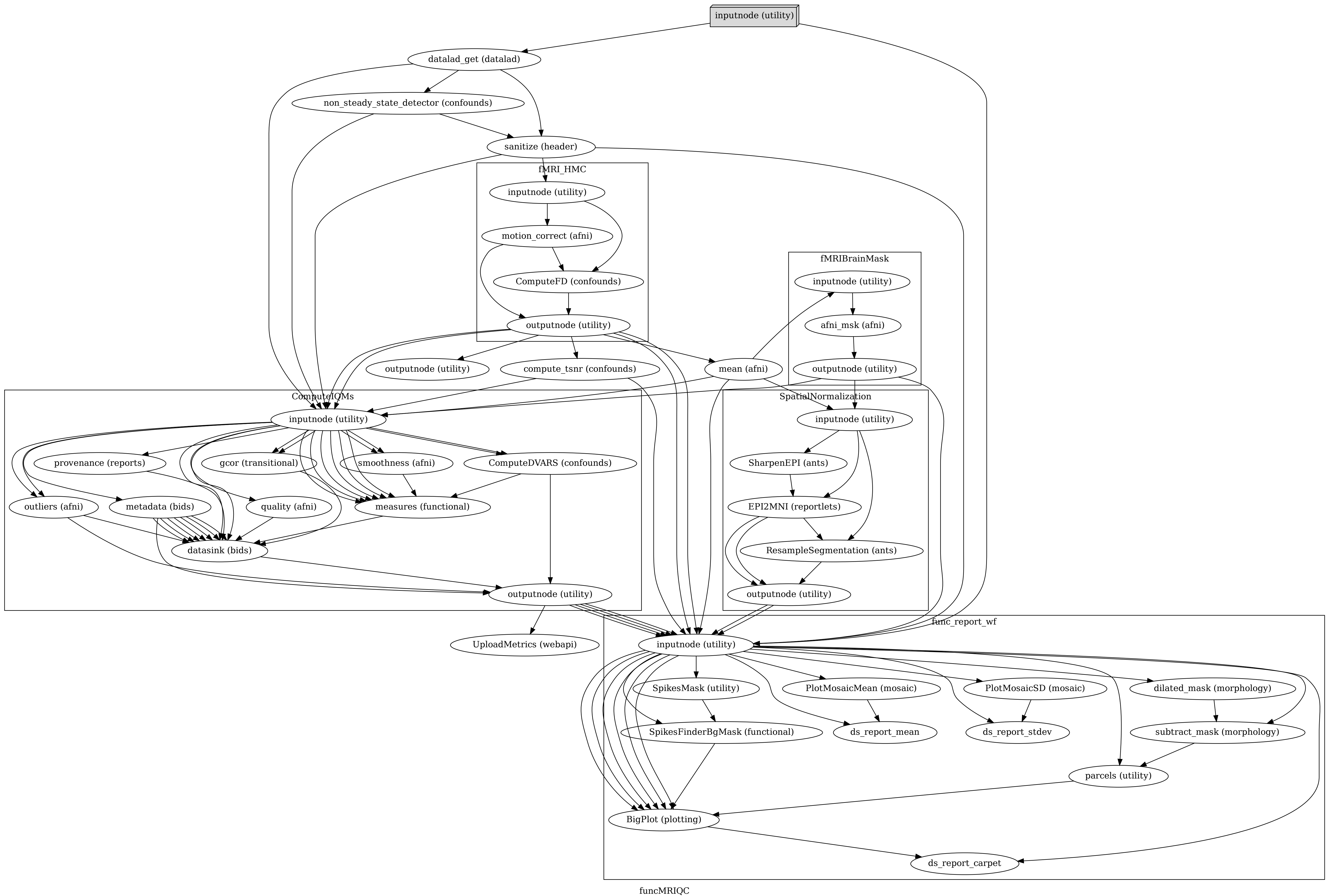
funcMRIQC
